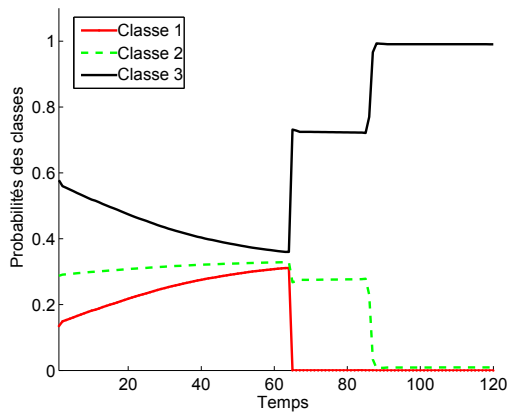
(a) Classification Bayésienne locale.
