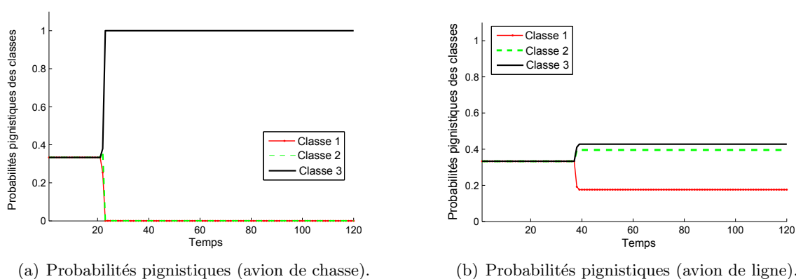
FIGURE 2.18: Effet des fausses associations sur la classification.
