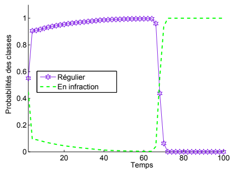
(a) Classification locale de l'objet 2 par le capteur 1.
