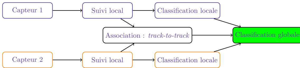
FIGURE 4.5: Organigramme de la solution proposée réduite au cas de deux capteurs.
