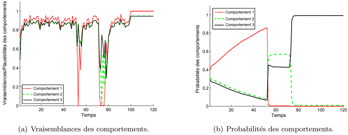
FIGURE 2.11: Classification Bayésienne basée sur les comportements de cibles aériennes (application 1).
