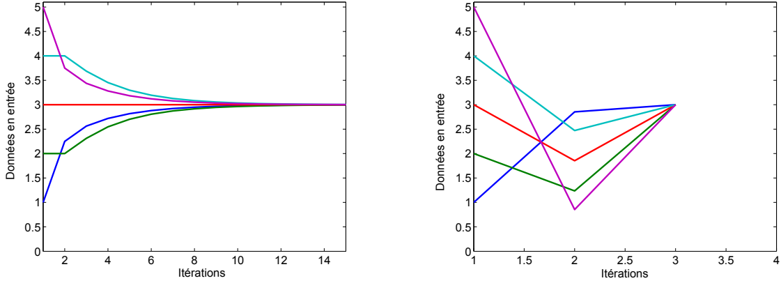
(a) Calcul de la valeur moyenne à l'aide du consensus asymptotique.
