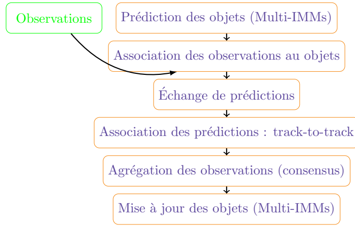
FIGURE 4.15: Étapes principales de l'algorithme de suivi distribué.
