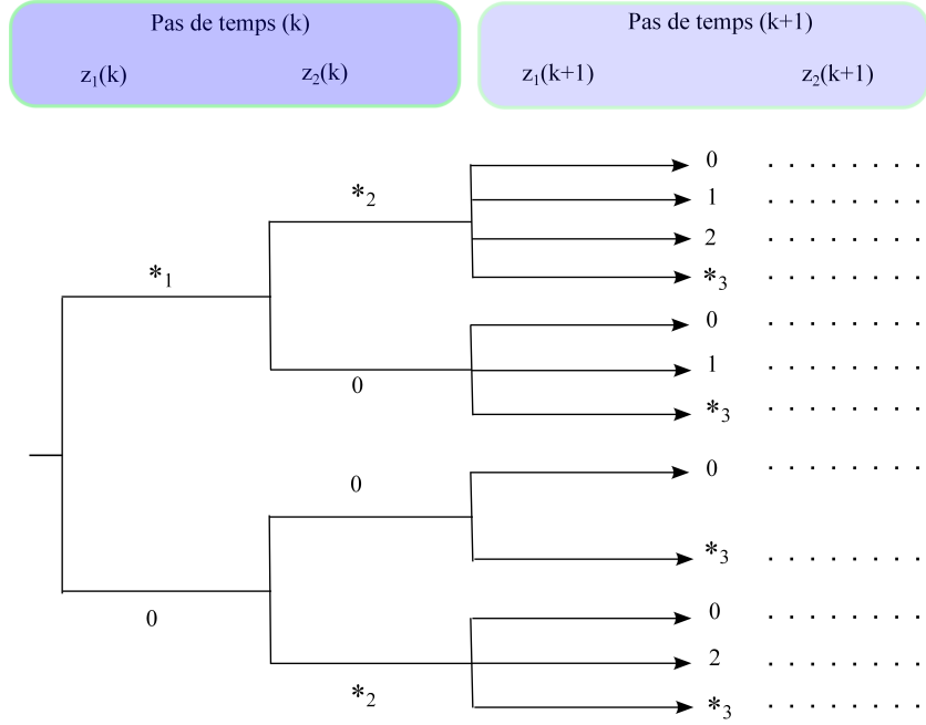
FIGURE 1.5: Génération d'hypothèses dans une méthode MHT .
