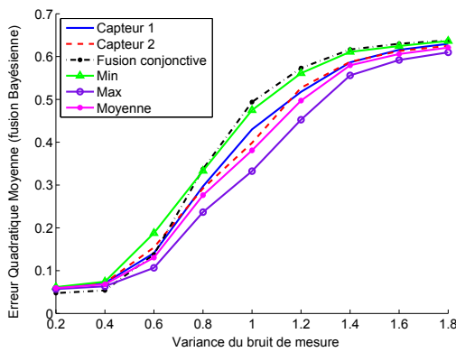
(a) Résultats, locaux et globaux, de la classification Bayésienne.
