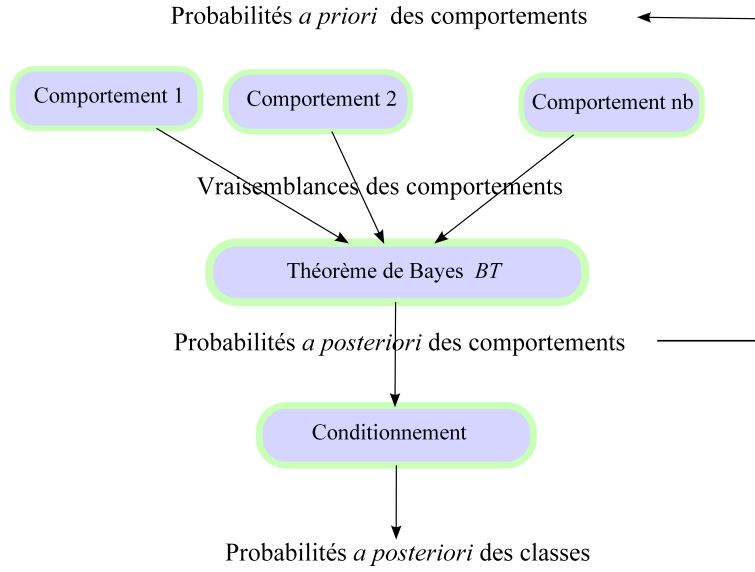
FIGURE 2.7: Organigramme du classifieur Bayésien.
