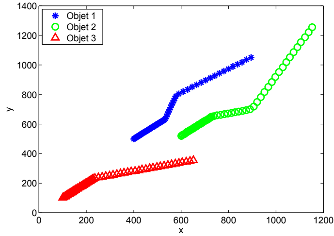
FIGURE 4.6: Scénario de 3 objets manœuvrants observés par deux capteurs peu fiables.
